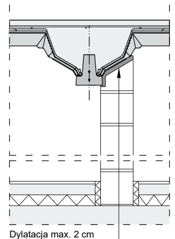
Dylatacja max. 2 cm wypełniona pianą poliuretanową lub wełną mineralną
