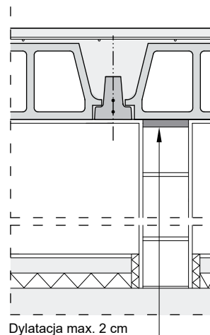
Dylatacja max. 2 cm wypełniona pianą poliuretanową lub wełną mineralną
