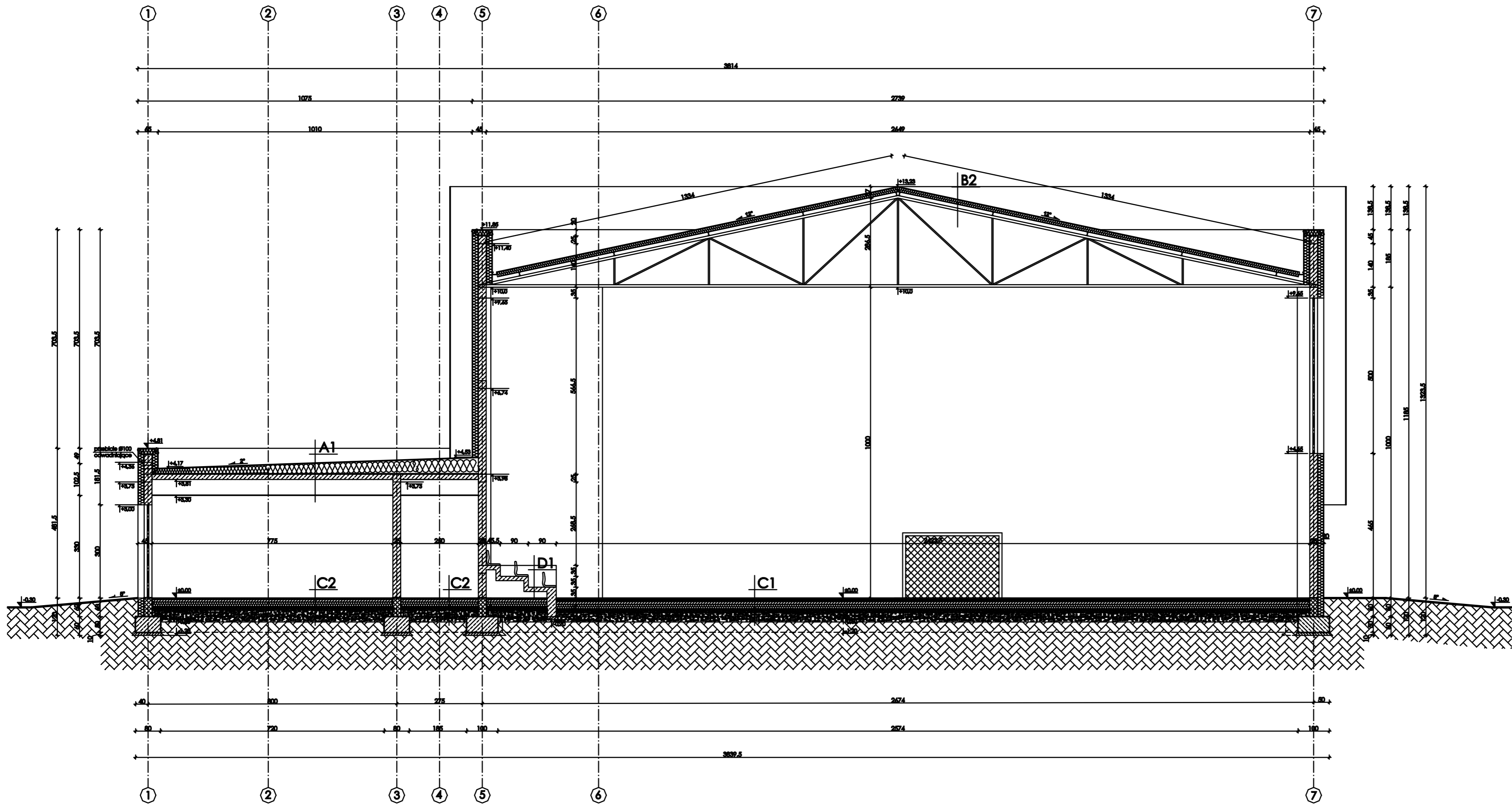
PRZEKRÓJ A-A skala 1:100
